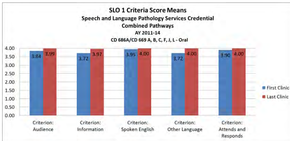
SLO 1 - CD 686A
